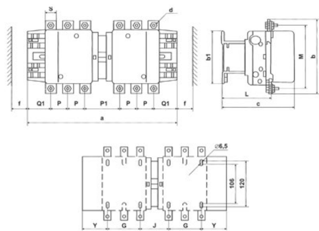
КТЭ rew 115 А; КТЭ rew 150 А; КТЭ rew 185 А; КТЭ rew 225 А; КТЭ rew 265 А; КТЭ rew 330 А
