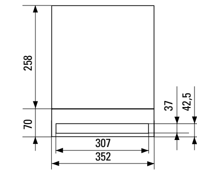
Вырез под рамку
