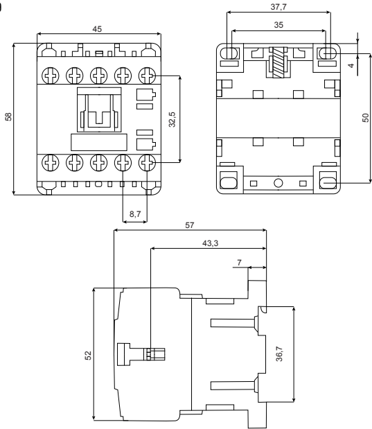
КМЭ 0910; КМЭ 1210; КМЭ 1810
