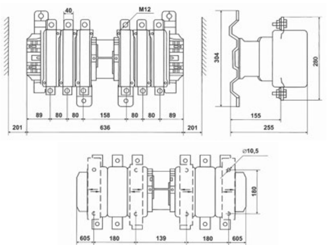
КТЭ rew 630 А
