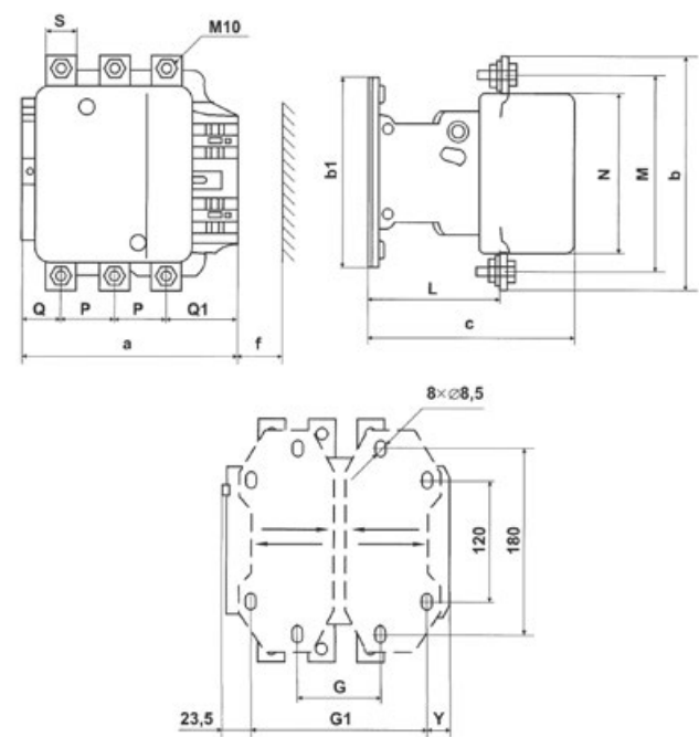
КТЭ-400 А; КТЭ-500 А
