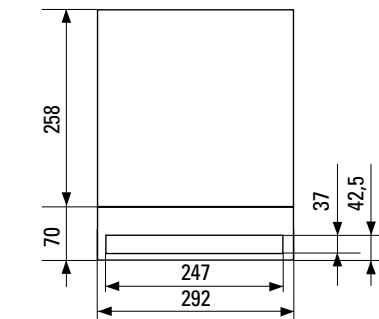
Вырез под рамку
