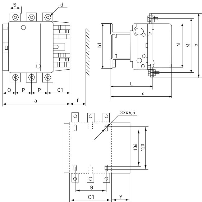
КТЭ-400 А; КТЭ-500 А
